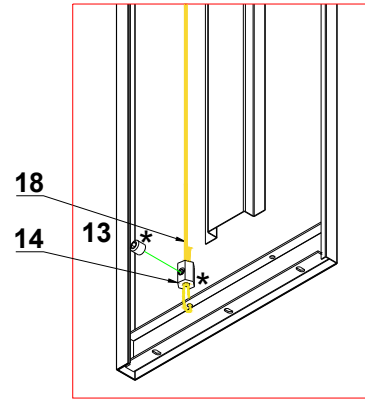
Detay B / Adım - 1 | Detail B / Step - 1 Деталь В / Этап - 1 | التفاصيل ب / الخطوة 1
