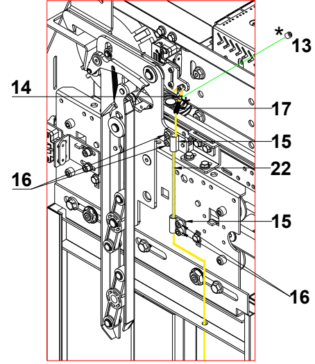
Detay B | Detail B Деталь В | التفاصيل ب
