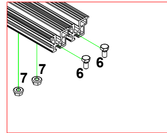
Detay A | Detail A Деталь А | تفصيل أ
