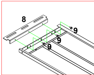
Panel Üst / Top Of The Panel Панель Верхняя | اللوحة العلوية
